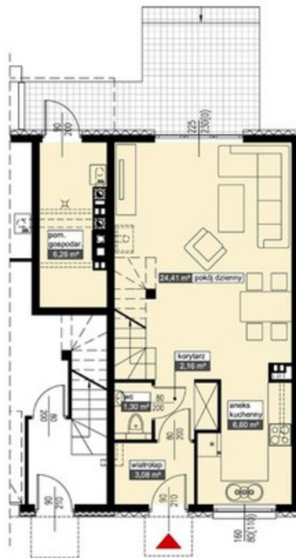
RZUT PARTERU
