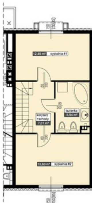
RZUT 1 PIĘTRA
