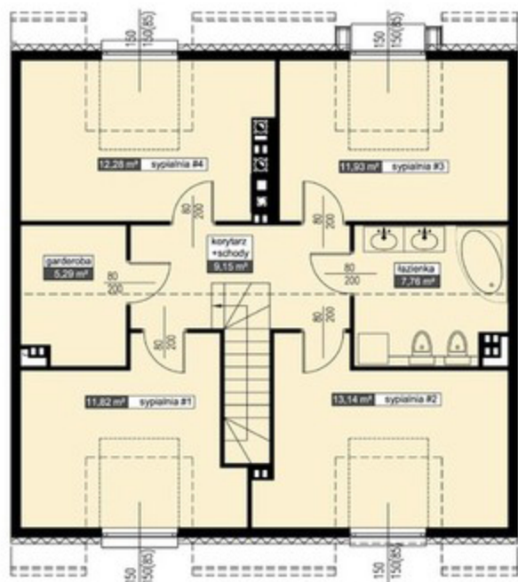
RZUT PODDASZA
