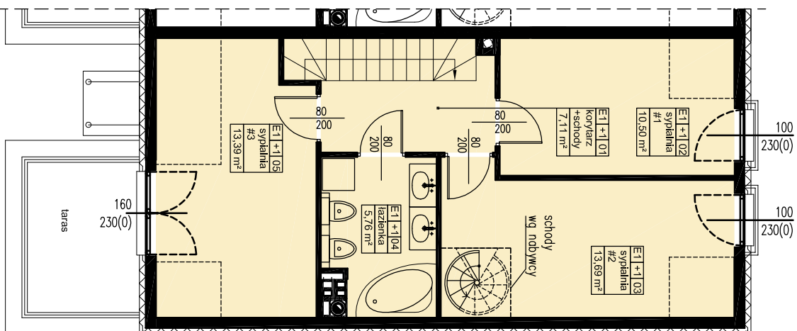
RZUT PODDASZA 1 PIĘTRO
